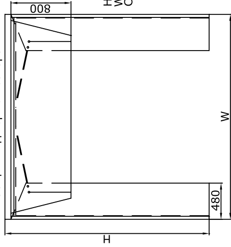
Общий вид герметизатора
